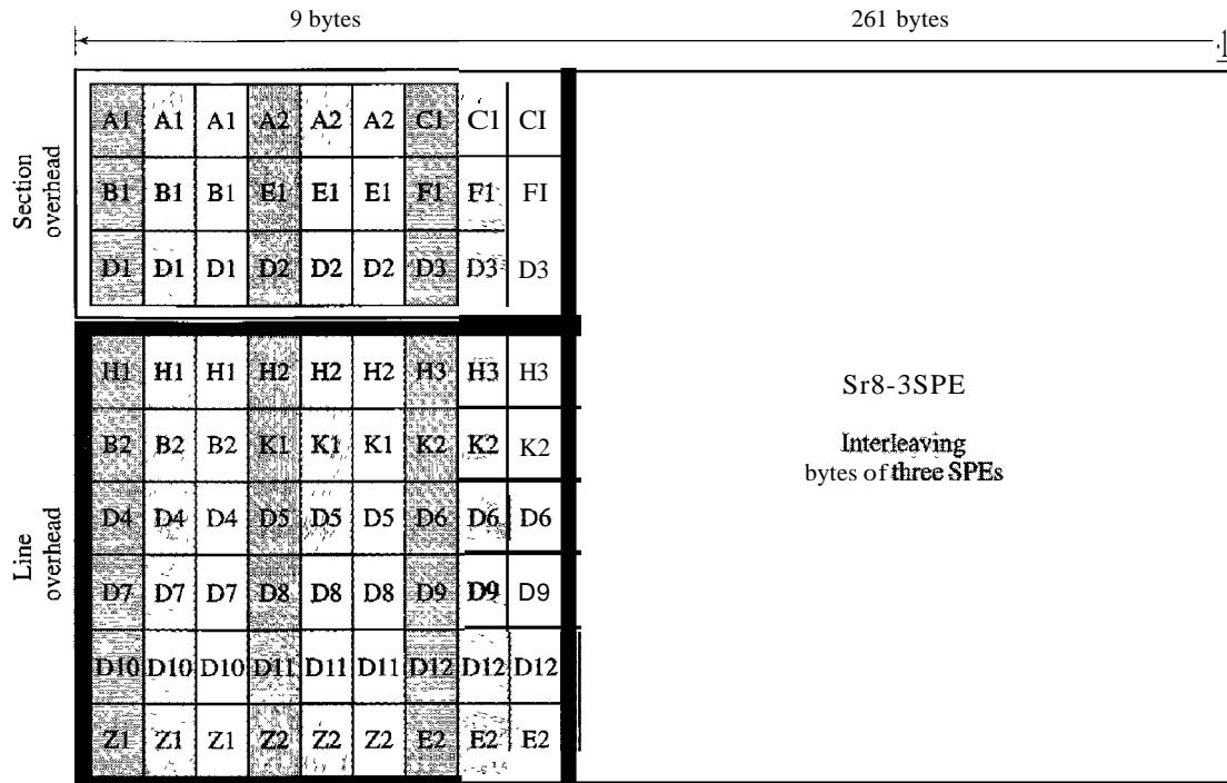
Figure 17.14 AnSTS-3frame
